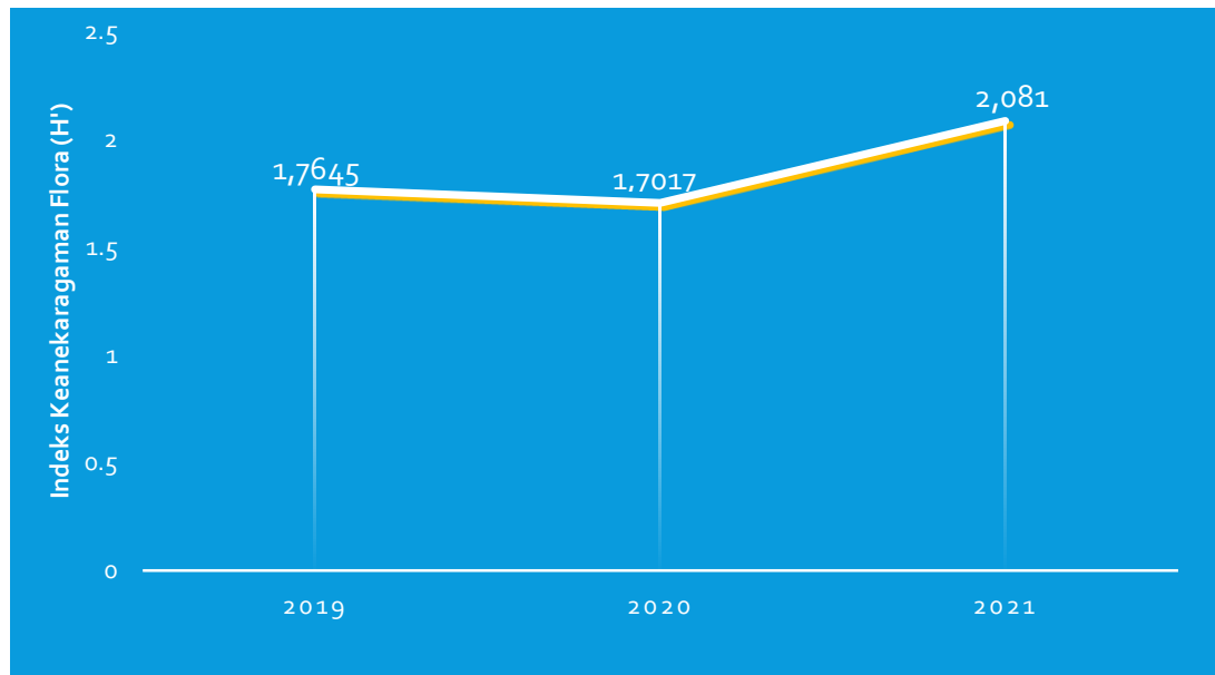
Gambar 1. Grafik perbandingan data nilai indeks keanekaragaman flora
