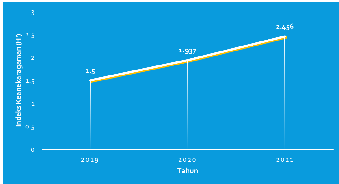
Gambar 2. Grafik perbandingan nilai indeks keanekaragaman Shannon-Wiener di SEGWWL dari tahun 2019-2021
